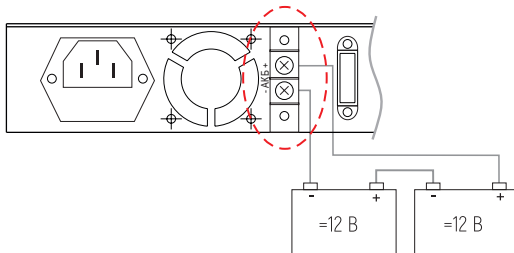
Рис. 11 Подключение двух последовательно соединенных АКБ напряжением 24 В, емкостью 17 А·ч (в двухзональных блоках емкостью 26 А·ч)
