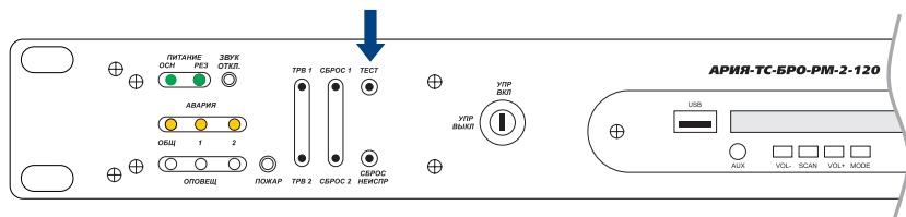
Рис. 46. Программирование сопротивления линий оповещения. Индикация режима «Неисправность»
