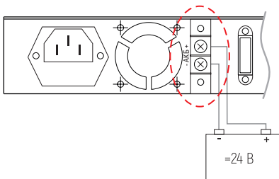
Рис. 10 Подключение одной АКБ напряжением 24 В, емкостью 17 А·ч (в двухзональных блоках емкостью 26 А·ч)
