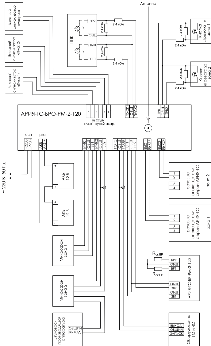
Рис. 44. Схема подключения внешнего оборудования к блоку речевого оповещения АРИЯ-ТС-БР-О-РМ-2-120
